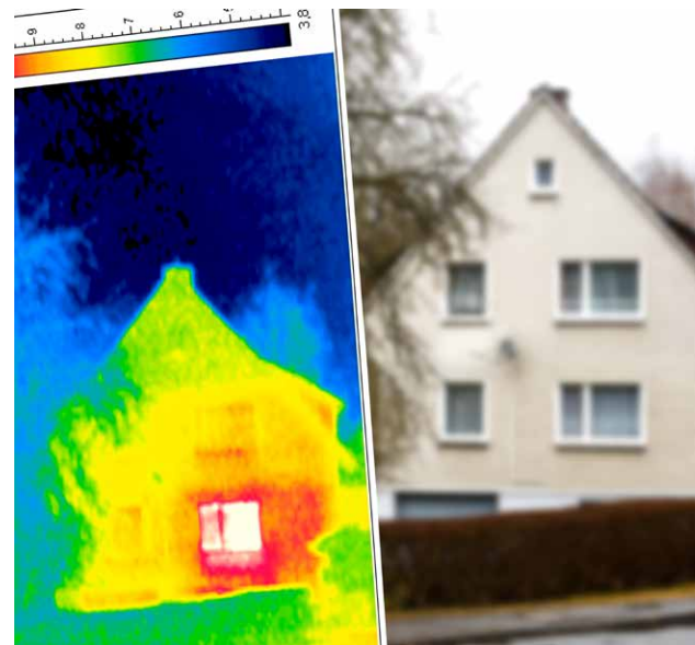
Beispiel Wärmeverlust am Fenster
